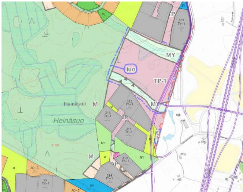
Kuva 2. Vt 4 yleissuunnitelman mukaiset valtatie ja rinnakkaisteiden linjat violetilla viivoituksella. Kuvassa näkyy myös voimassa oleva osayleiskaava sekä voimassa olevat asemakaavat.
